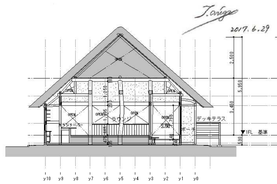
断面図 S = 1 / 100
